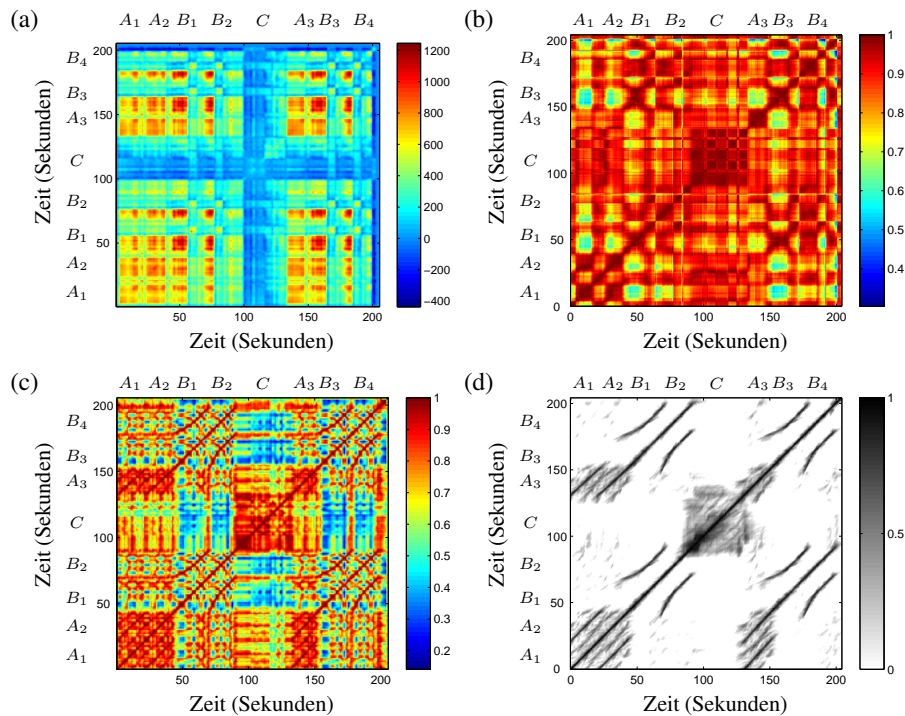
Abbildung 3: Selbstähnlichkeitsmatrizen für die in Abbildung 2 dargestellten Merkmale: (a) MFCC-basierte Merkmale, (b) Tempo-basierte Merkmale, (c) Chroma-basierte Merkmale. (d) zeigt eine strukturell verbesserte Version der Selbstähnlichkeitsmatrix aus (c).
