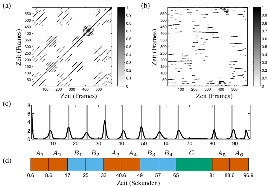
Abbildung 5: Novelty-basierte Segmentierung auf Strukturmerkmalen für eine Aufnahme der Mazurka Op. 24, No. 1 von Frédéric Chopin. (a) Selbstähnlichkeitsmatrix basierend auf Chromamerkmale. (b) Zeit-Lag Matrix. (c) Novelty-Kurve. (d) Manuelle Annotation der musikalischen Form der Aufnahme.
