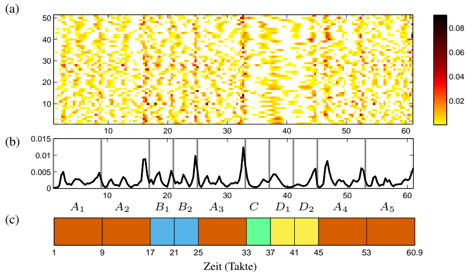
Abbildung 6: Cross-Version Strategie für Tempo-basierte Segmentierung am Beispiel von der Mazurka Op. 68, No. 3 von Chopin (aus [MPD12]). (a) Farbkodierte Novelty-Kurven für 51 Aufnahmen (mit transformierten Zeitachsen). (b) Versionsübergreifende Novelty-Kurve. (c) Manuelle Annotation der musikalische Form.
