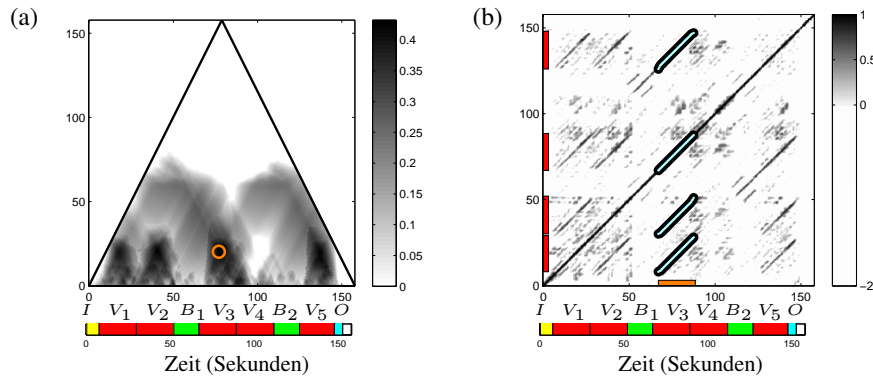
Abbildung 4: (a) Scape-Plot zum Beatles-Song “You Can’t Do That.” (b) Selbstähnlichkeitsmatrix mit Thumbnail (in orange, horizontale Achse) und allen zum Thumbnail in Beziehung stehenden Segmenten (in rot, vertikale Achse), die in Form einer sogenannten Pfadfamilie (in cyan) erfasst werden.
